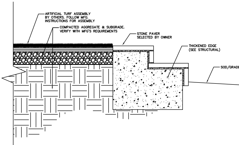
DETAIL A SCALE: 3/4" = 1'-0"
