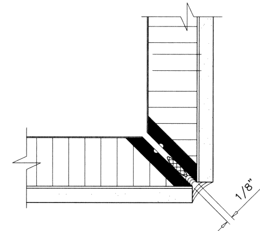
QUIRK MITER EDGE
