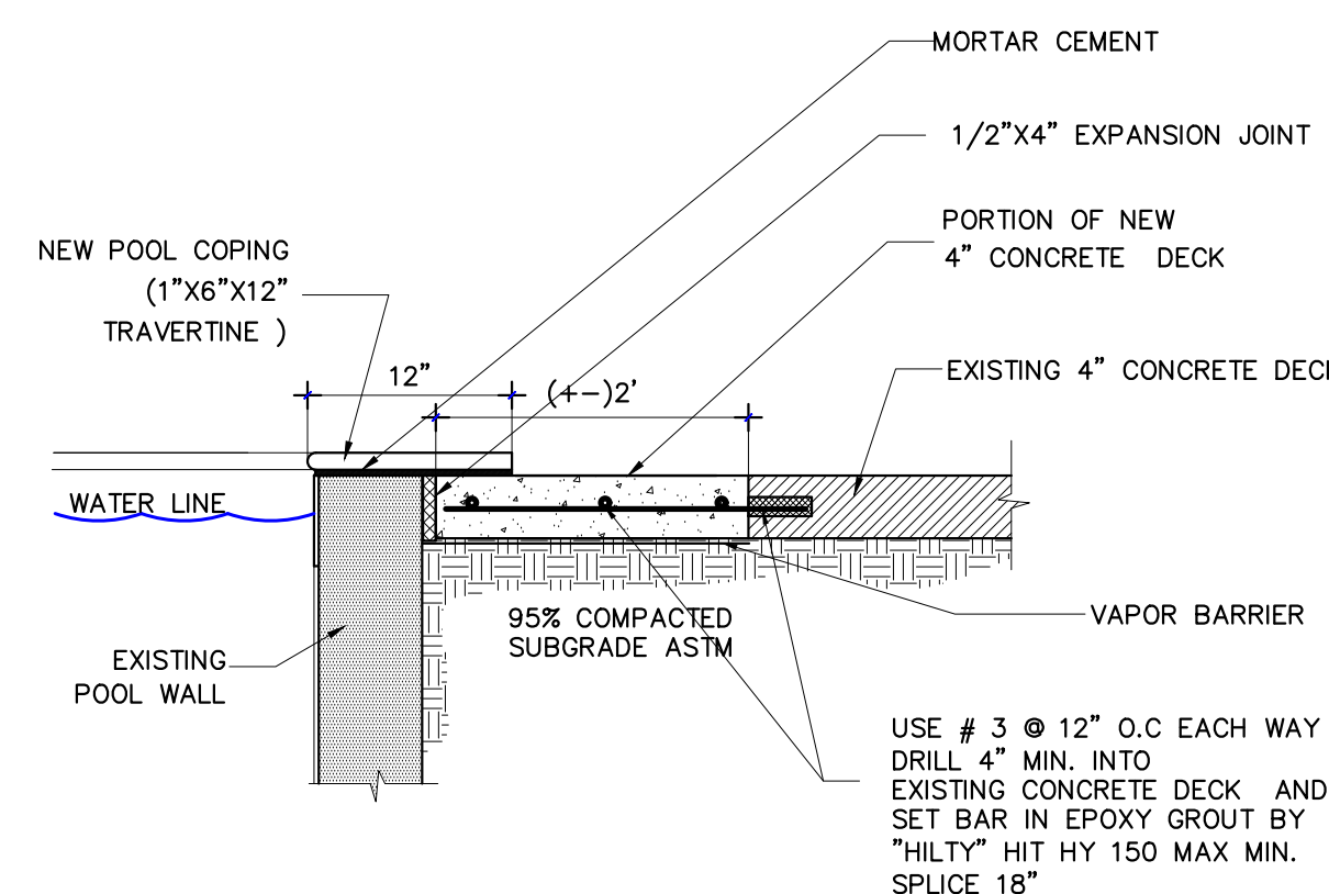
POOL DECK REPAIR DETAIL scale: N.T.S
