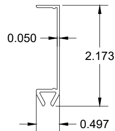
7 JAMB SEAL
