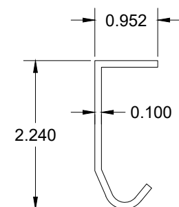
9 DOOR TRACK (2" OPT.)
