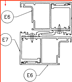
STD. INTERLOCK
