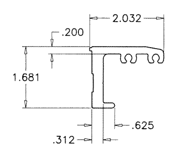
E10 CORNER BLOCK
