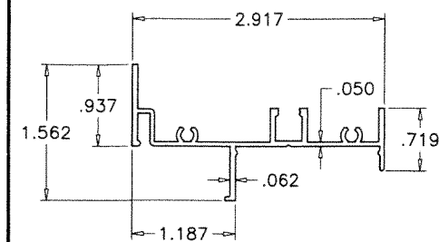
E1 FRAME
