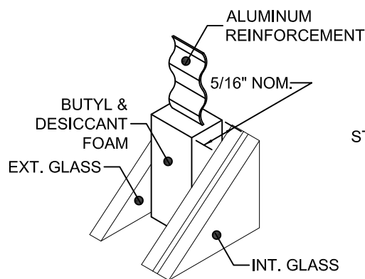
102 DURASEAL ® SPACER
