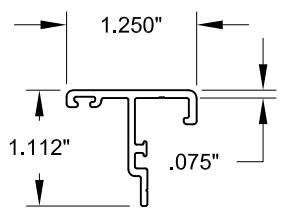
12 ASTRAGAL
