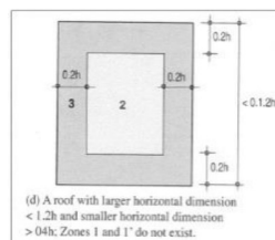
Roof zone layout (d)
