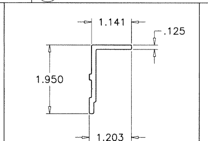
E18 CLOSURE DOOR STOP
