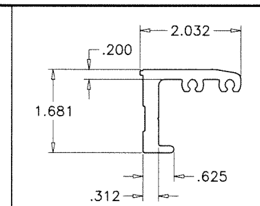
E10 CORNER BLOCK
