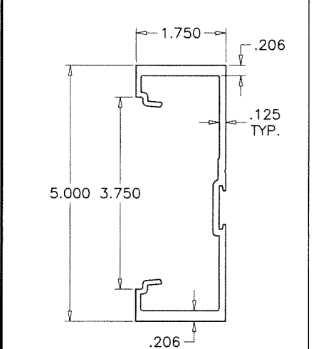
E35 TRANSOM JAMB (ES-8000)
