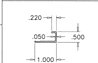
E37 DOOR STOP COVER
