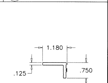
E17 DOOR SWEEP
