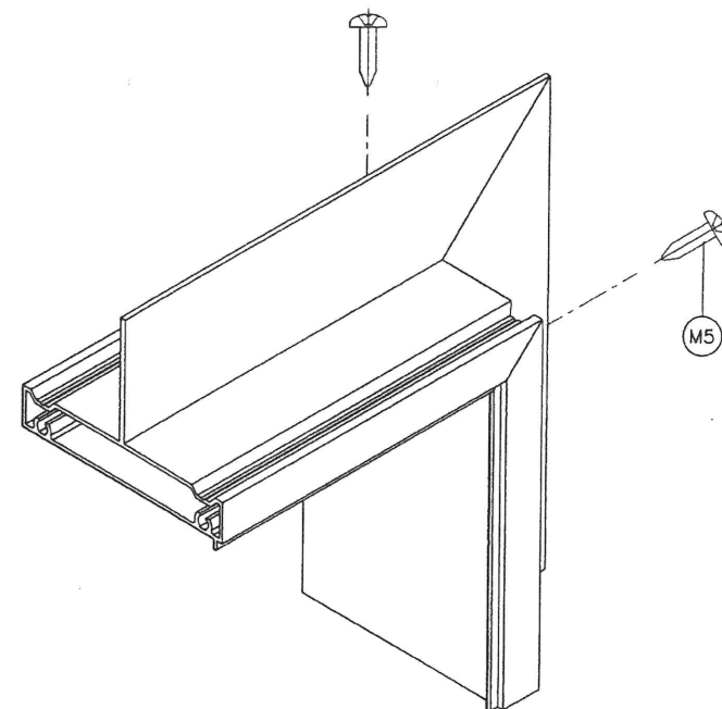
FIN FRAME ADAPTER CORNER
