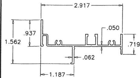
E1 FRAME
