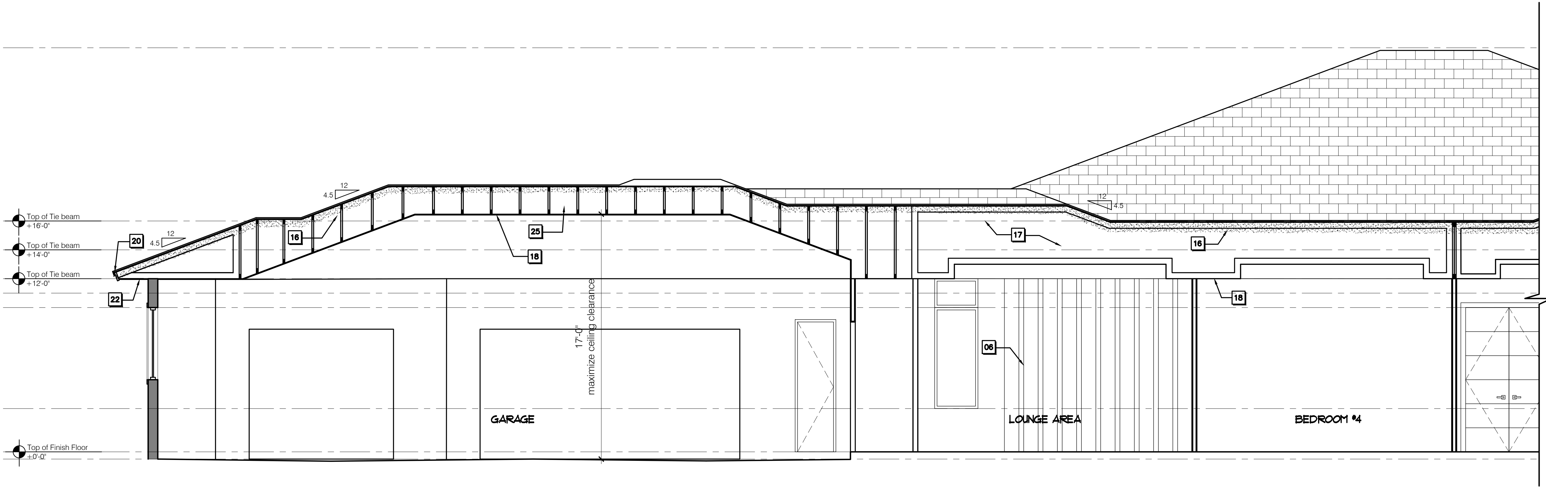
SECTION E 1/4" SCALE.
