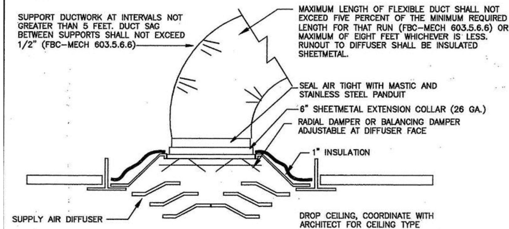
SUPPLY AIR DIFFUSER N.T.S. M\CD-1
