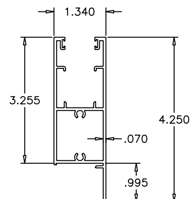
E21 TOP/BOTTOM HORIZ (OPTIONAL)
