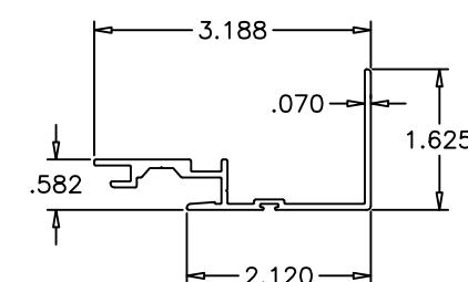
E15 POCKET HOOK
