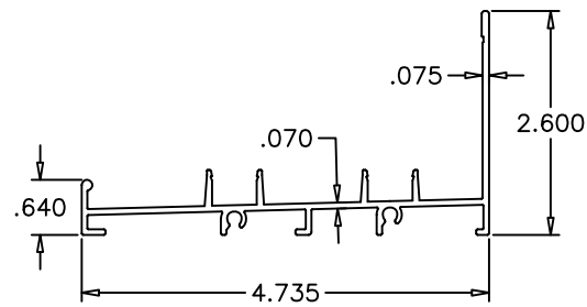
E1 FRAME SILL (2 TRACK)
