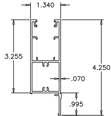
E7 TOP/BOTTOM HORIZ
