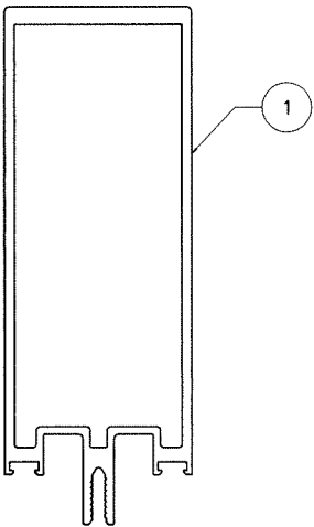
JAMB 'J1' MULLION 'M1'
