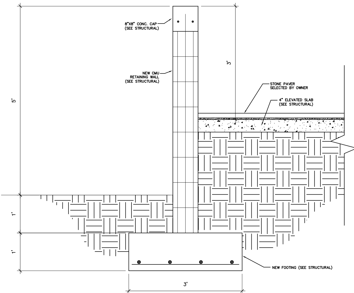
DETAIL C SCALE: 3/4" = 1'-0"
