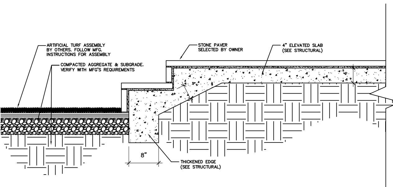
DETAIL B SCALE: 3/4" = 1'-0"
