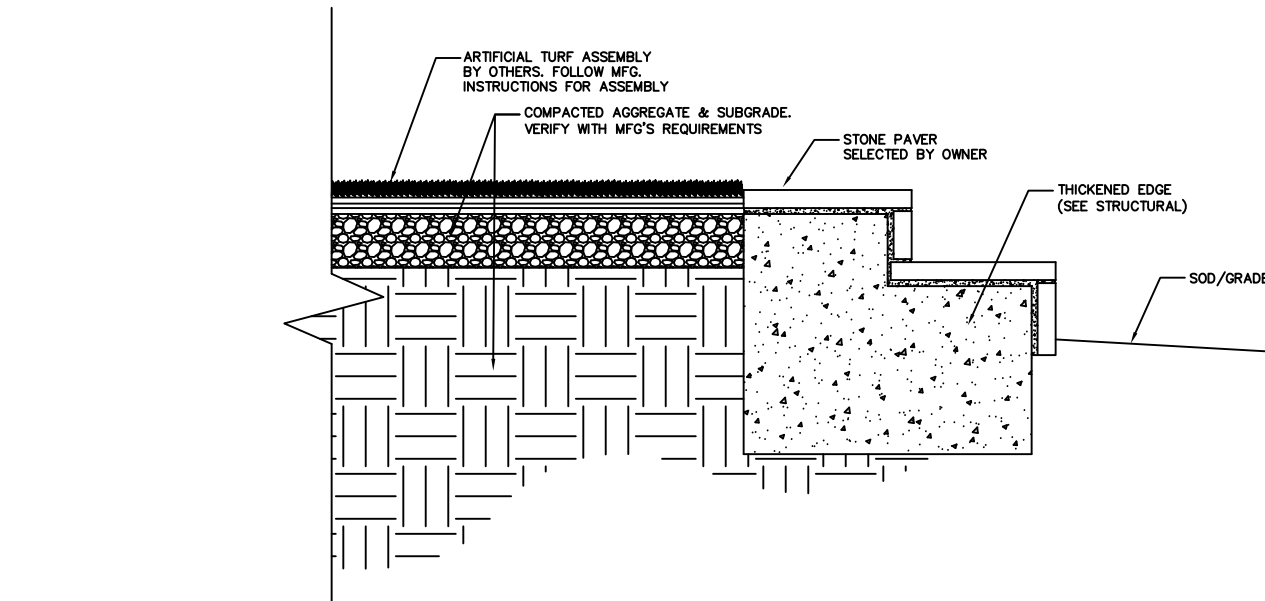
DETAIL A SCALE: 3/4" = 1'-0"
