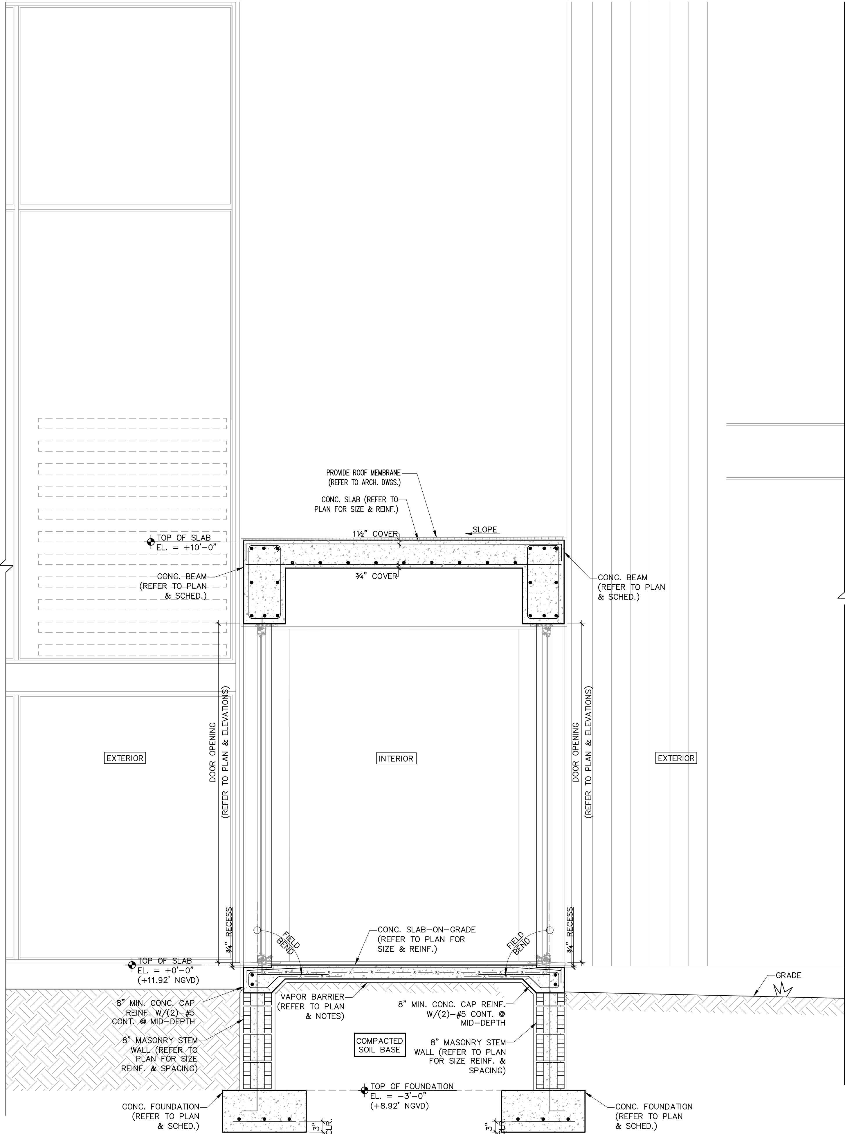
SECTION 3 SCALE : 3/4"=1'-0"
