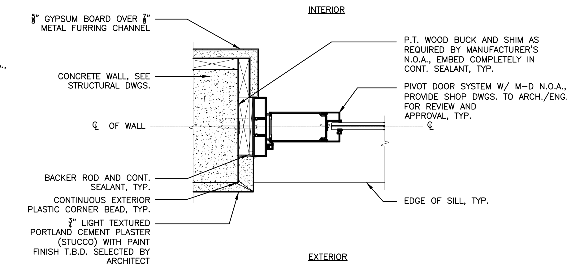
1 A-504 DOOR JAMB DETAIL - PIVOT DOOR SCALE: 3"=1'-0"
