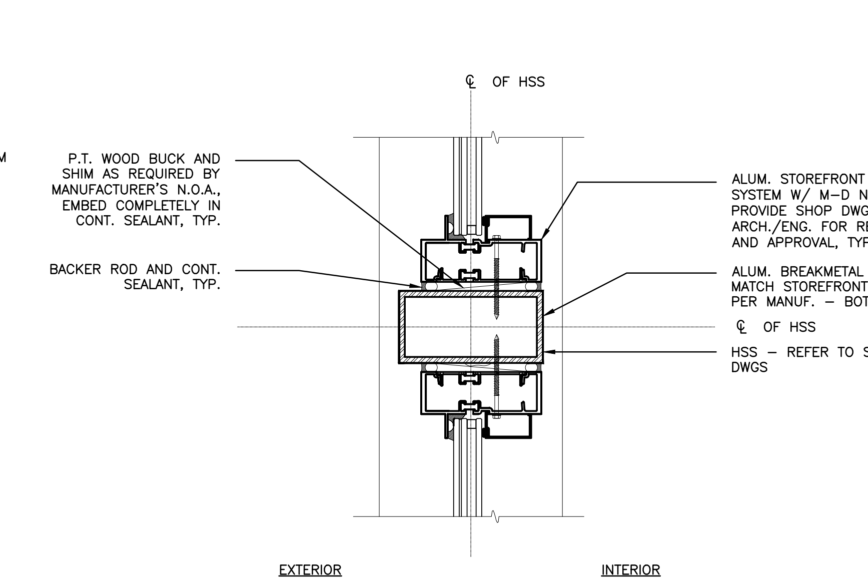
6 A-504 STOREFRONT - JAMB DETAIL @ TUBE STEEL SCALE: 3"=1'-0"
