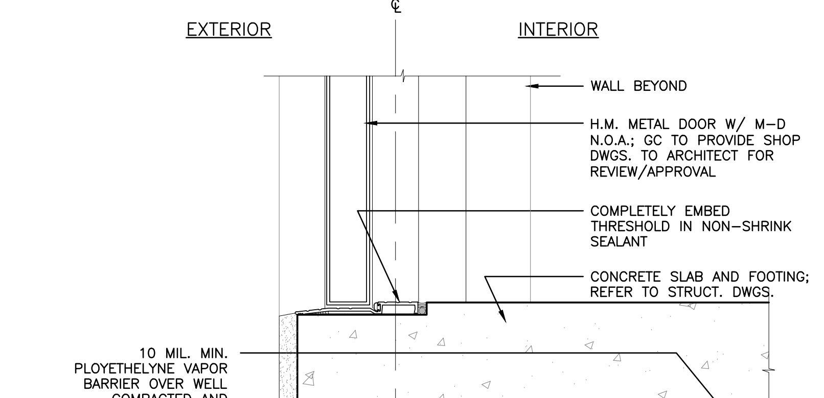
16 A-504 H.M. DOOR SILL DETAIL SCALE: 3"=1'-0"
