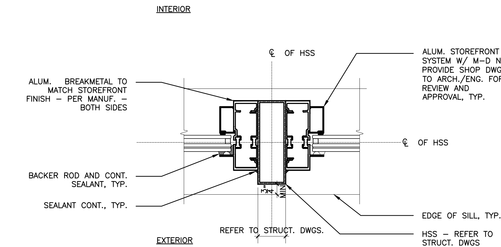
5 A-504 STOREFRONT - JAMB DETAIL @ TUBE STEEL SCALE: 3"=1'-0"
