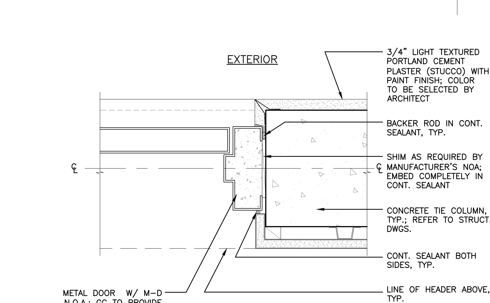
17 A-504 H.M. DOOR JAMB DETAIL SCALE: 3"=1'-0"
