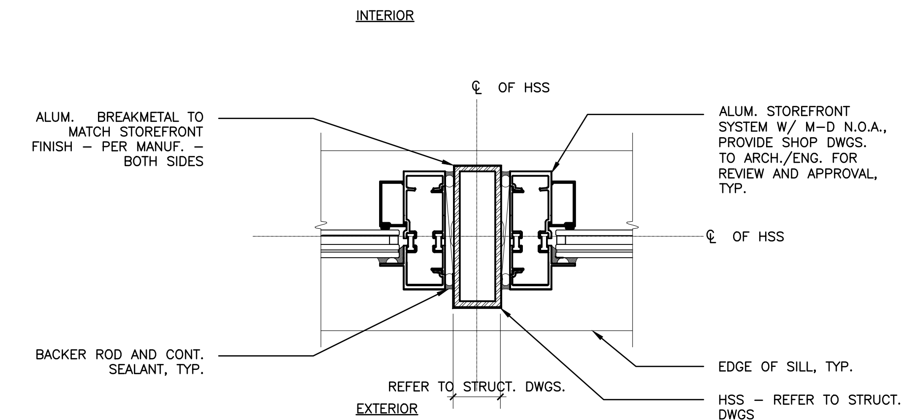
9 A-504 STOREFRONT - JAMB DETAIL @ TUBE STEEL SCALE: 3"=1'-0"
