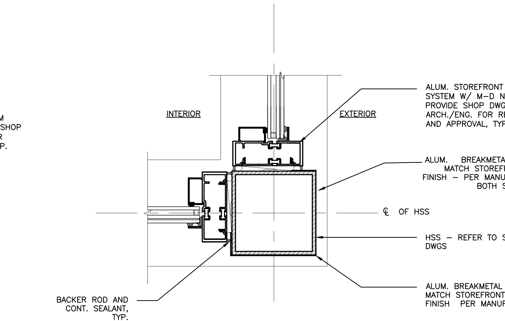
7 A-504 STOREFRONT - JAMB DETAIL (CORNER) SCALE: 3"=1'-0"
