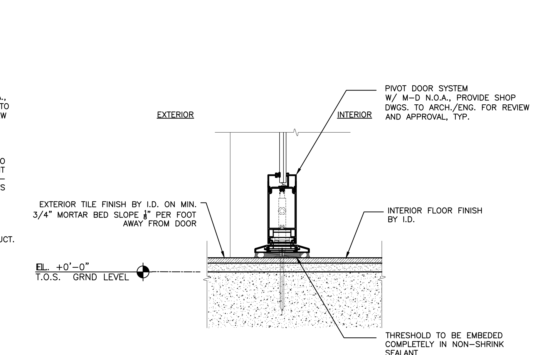
3 A-504 DOOR SILL DETAIL - PIVOT DOOR SCALE: 3"=1'-0"
