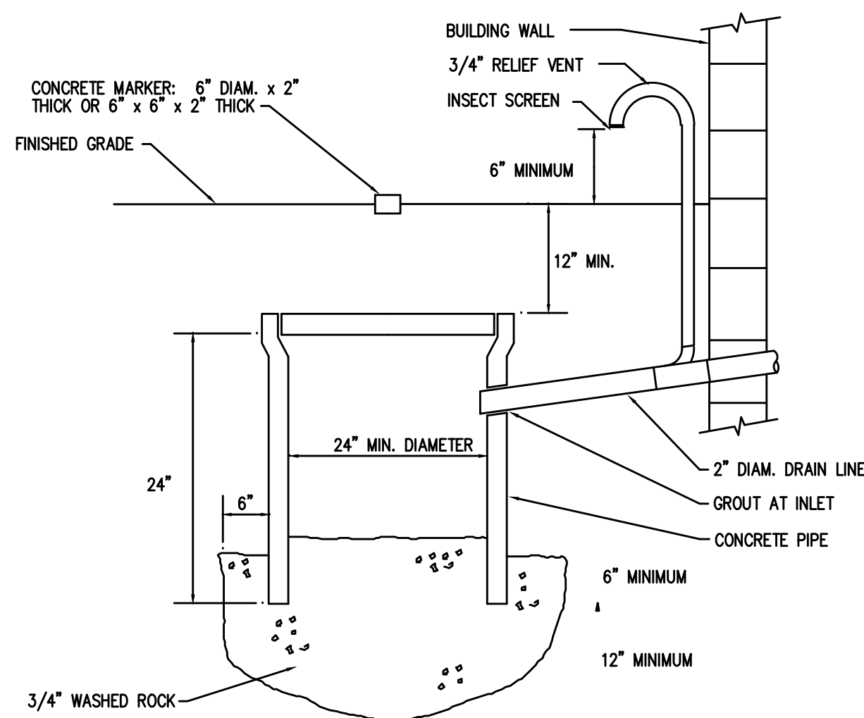
CONDENSATE DRYWELL DETAIL N.T.S.
