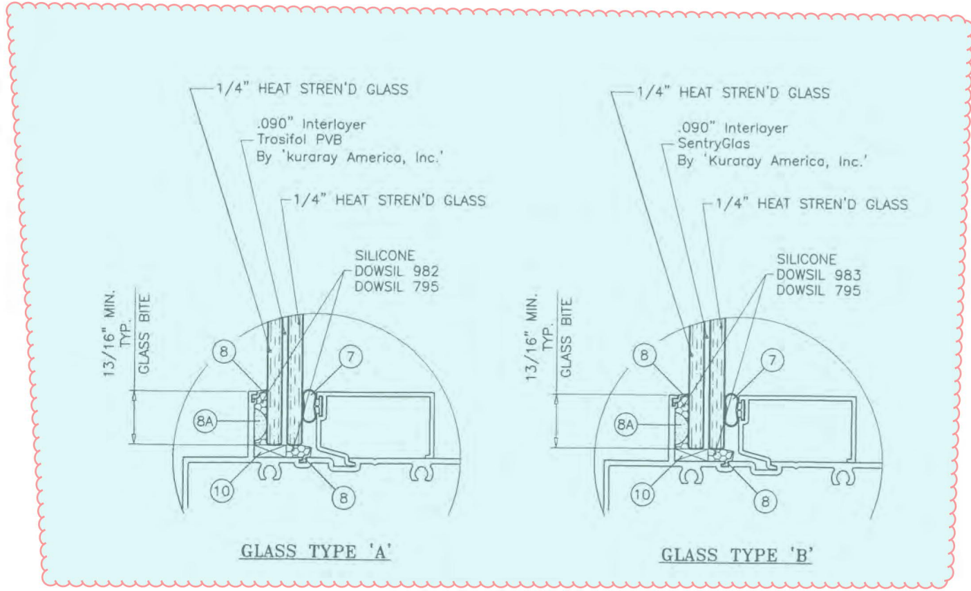
GLAZING OPTIONS
