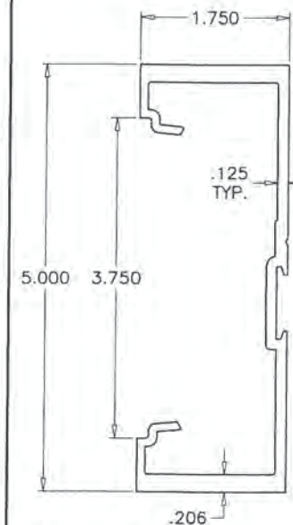
DOOR MULLION
