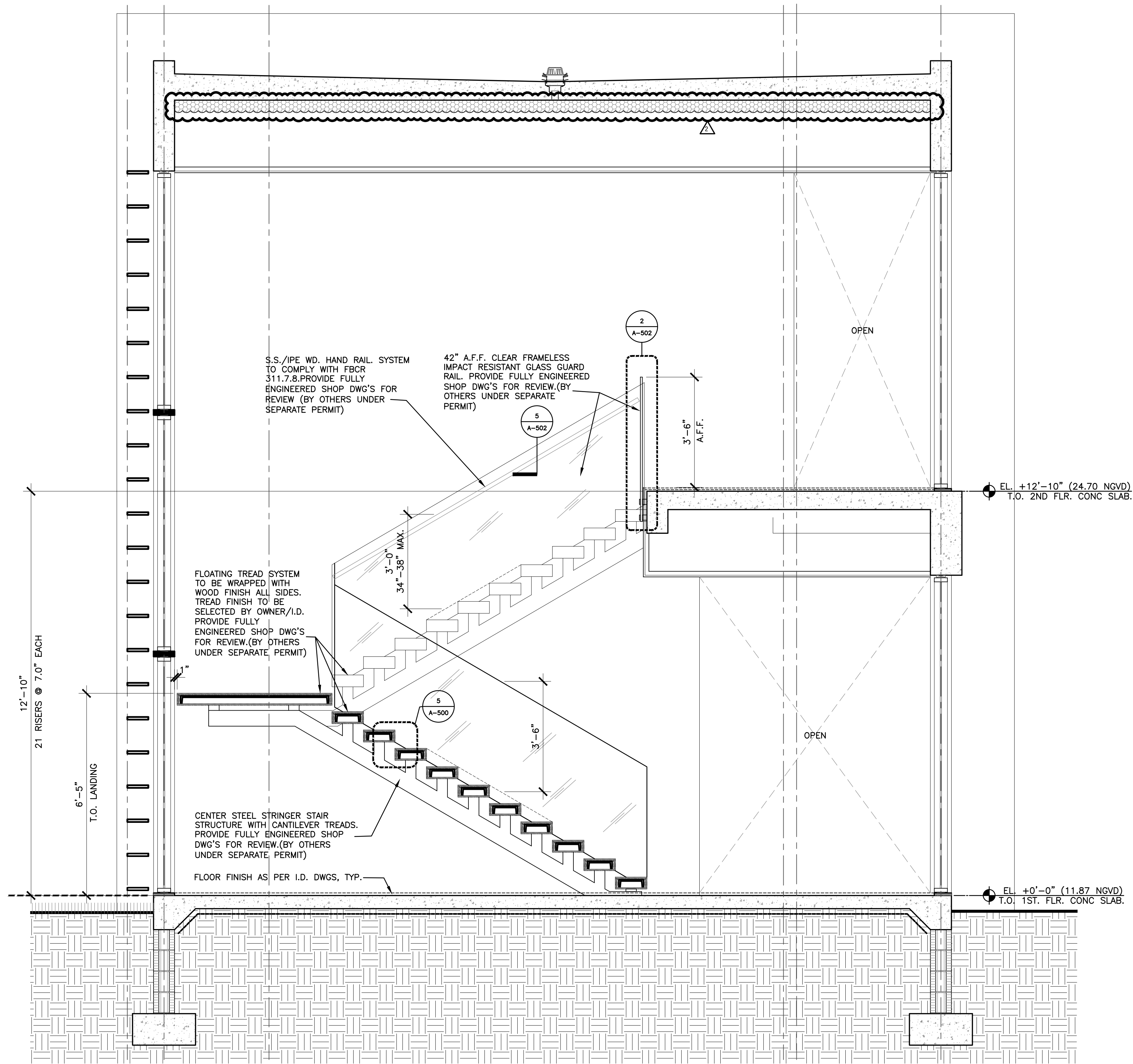
3 STAIR SECTION A-410 SCALE: 1/2"=1'-0"
