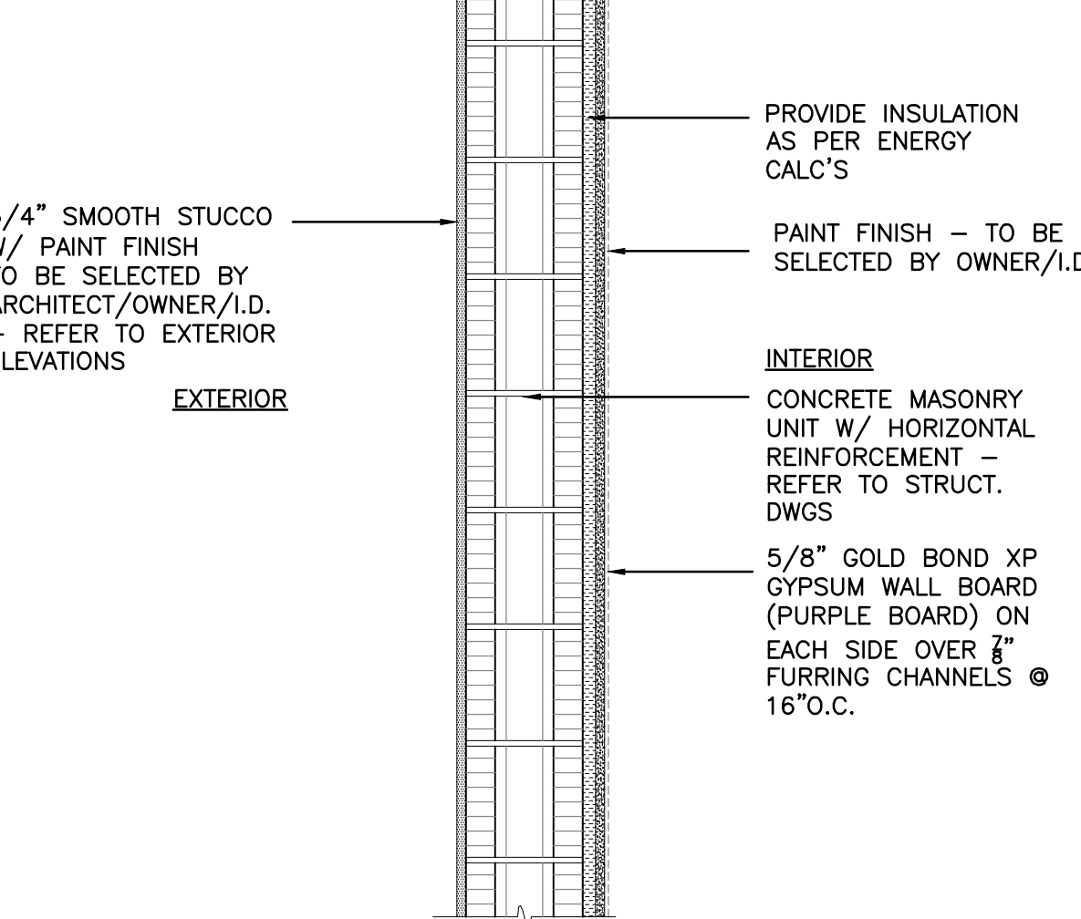
1 A-602 MASONRY - M1 SCALE: 1"=1'-0"
