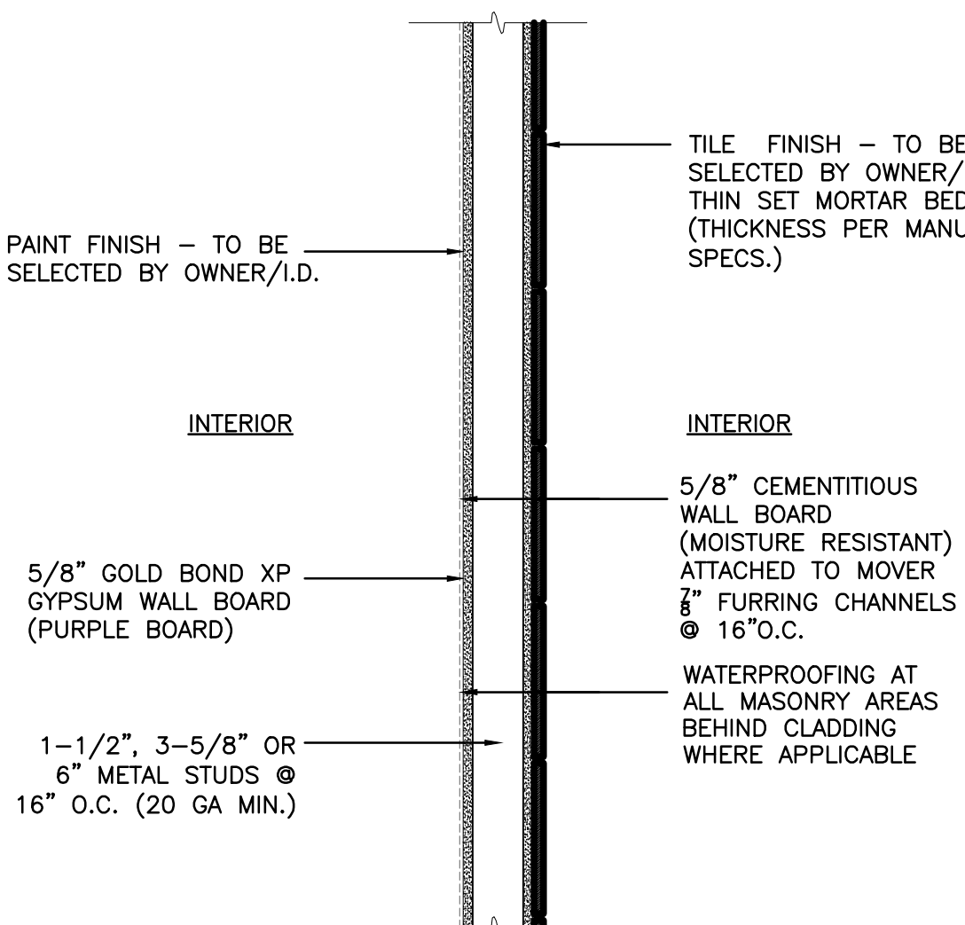
11 A-602 PARTITION - P2 SCALE: 1"=1'-0"
