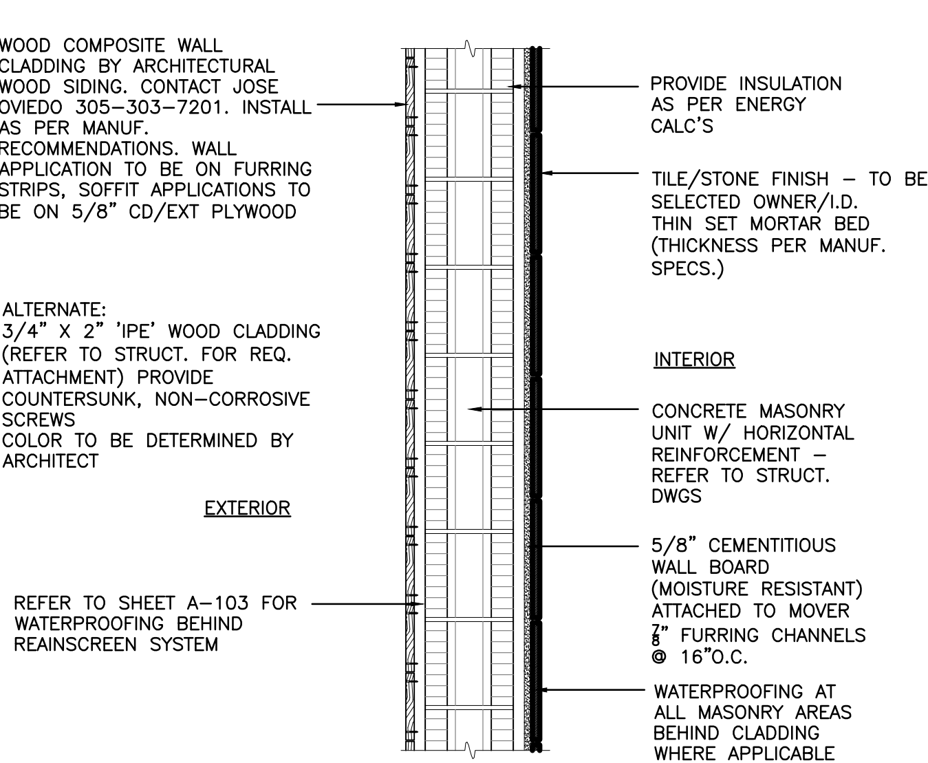
7 A-602 MASONRY - M7 SCALE: 1"=1'-0"
