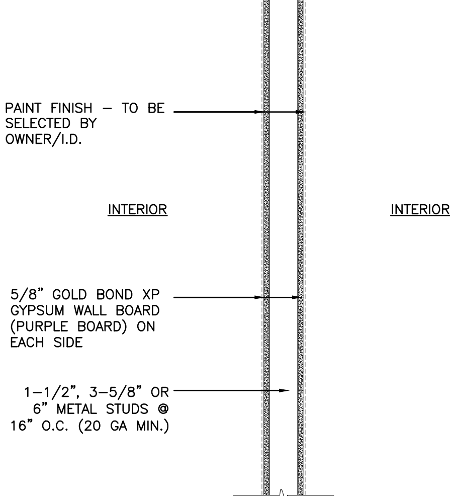
10 A-602 PARTITION - P1 SCALE: 1"=1'-0"
