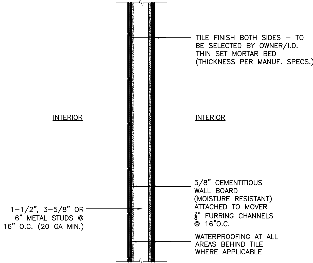
11 A-602 PARTITION - P2 SCALE: 1"=1'-0"
