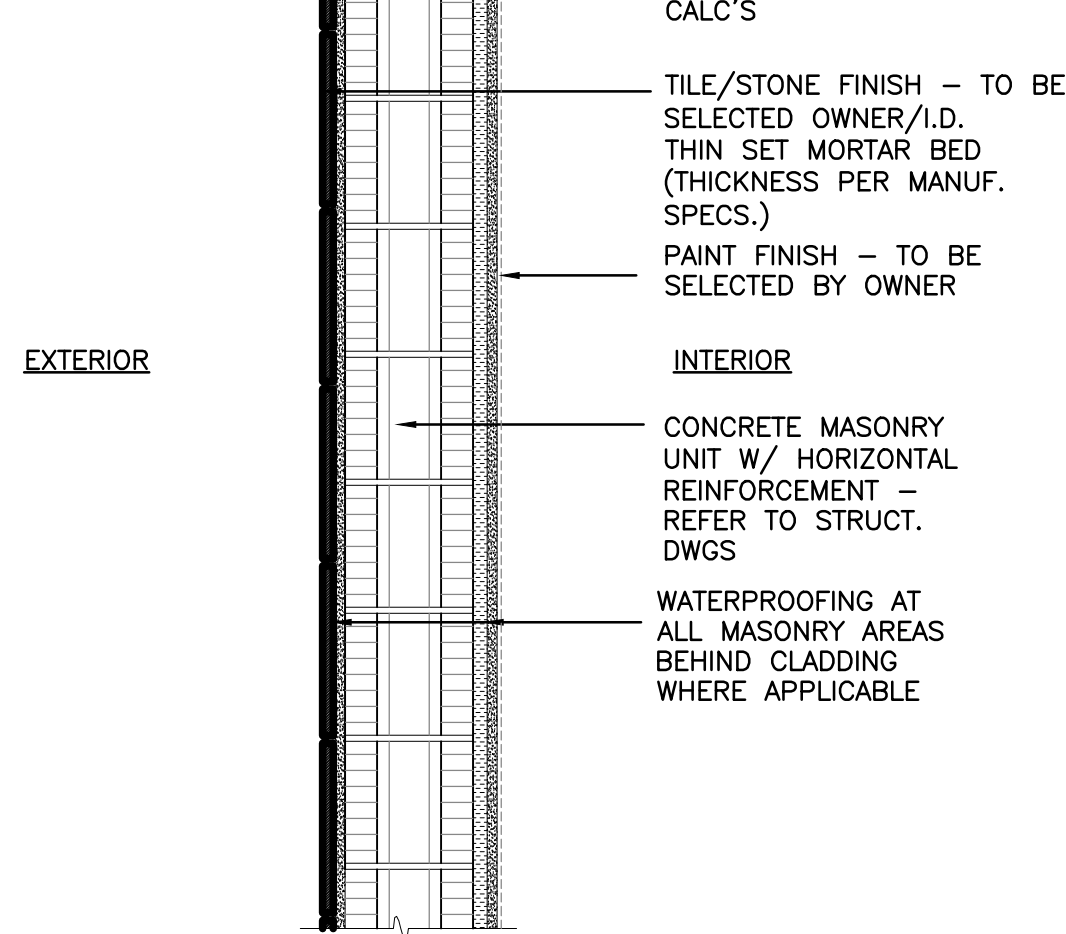
5 A-602 MASONRY - M5 SCALE: 1"=1'-0"
