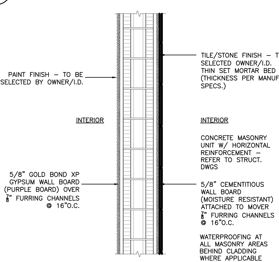
4 A-602 MASONRY - M4 SCALE: 1"=1'-0"
