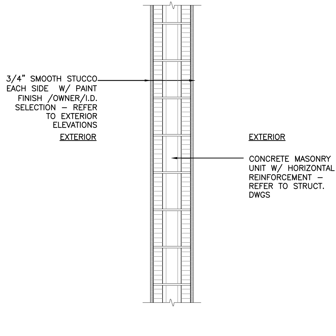
1 A-602 MASONRY - M1 SCALE: 1"=1'-0"
