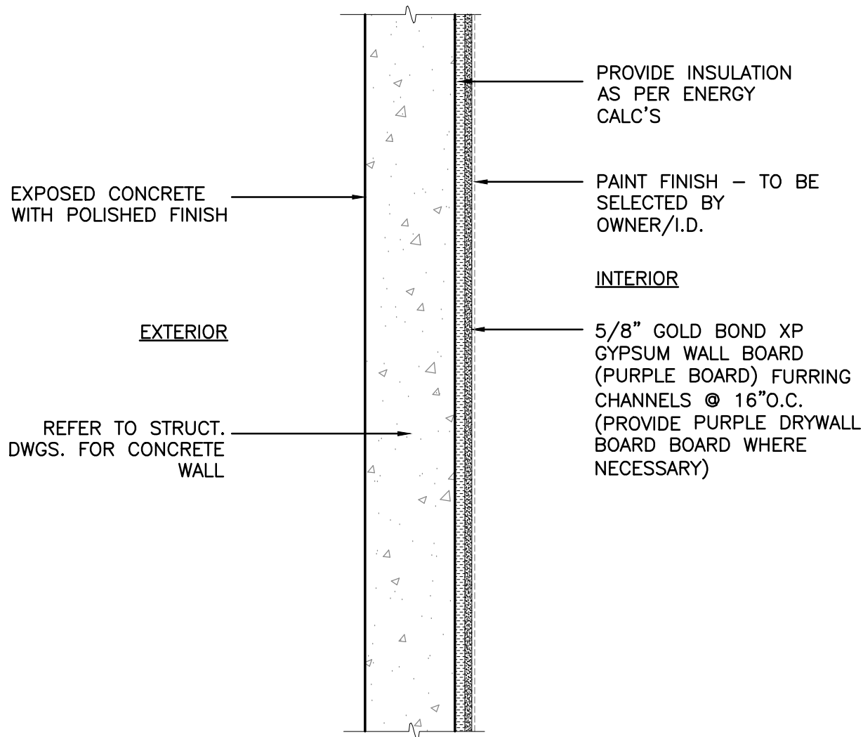
14 A-602 CONCRETE - C2 SCALE: 1"=1'-0"
