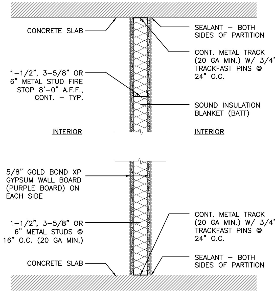
9 A-602 PARTITION-WALL TYP. SCALE: 1"=1'-0"
