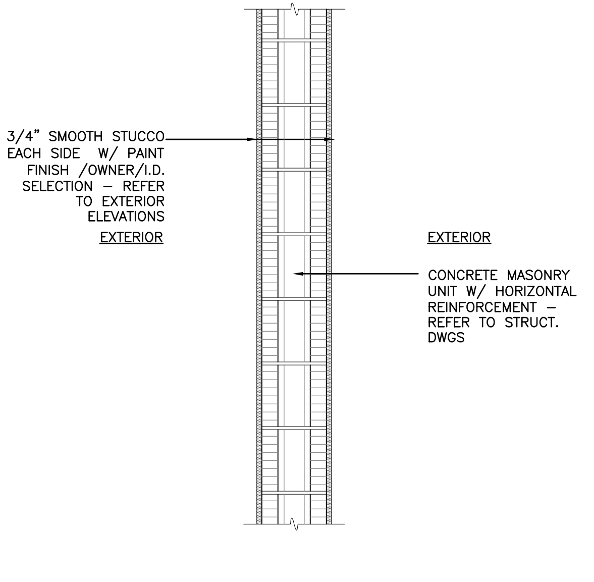
1 A-602 MASONRY - M1 SCALE: 1"=1'-0"
