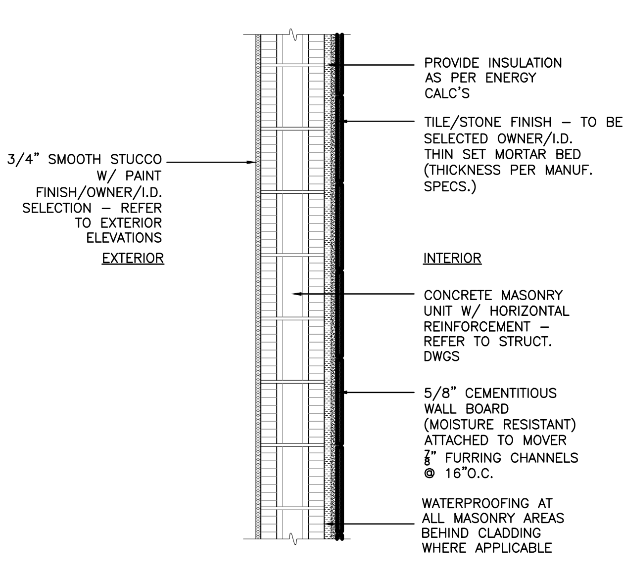
5 A-602 MASONRY - M5 SCALE: 1"=1'-0"
