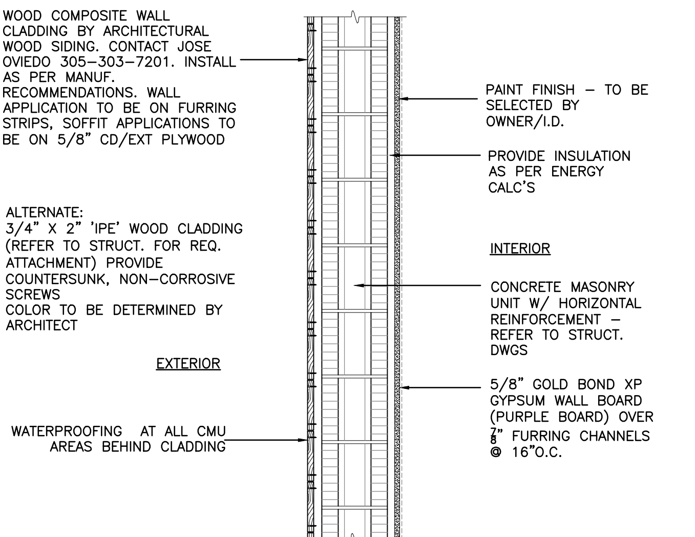
8 A-602 MASONRY - M8 SCALE: 1"=1'-0"
