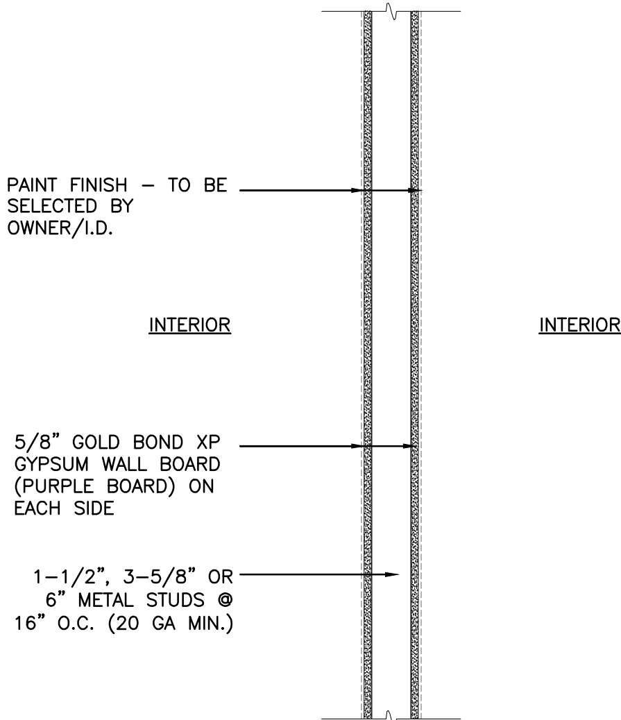
9 A-602 PARTITION-WALL TYP. SCALE: 1"=1'-0"
