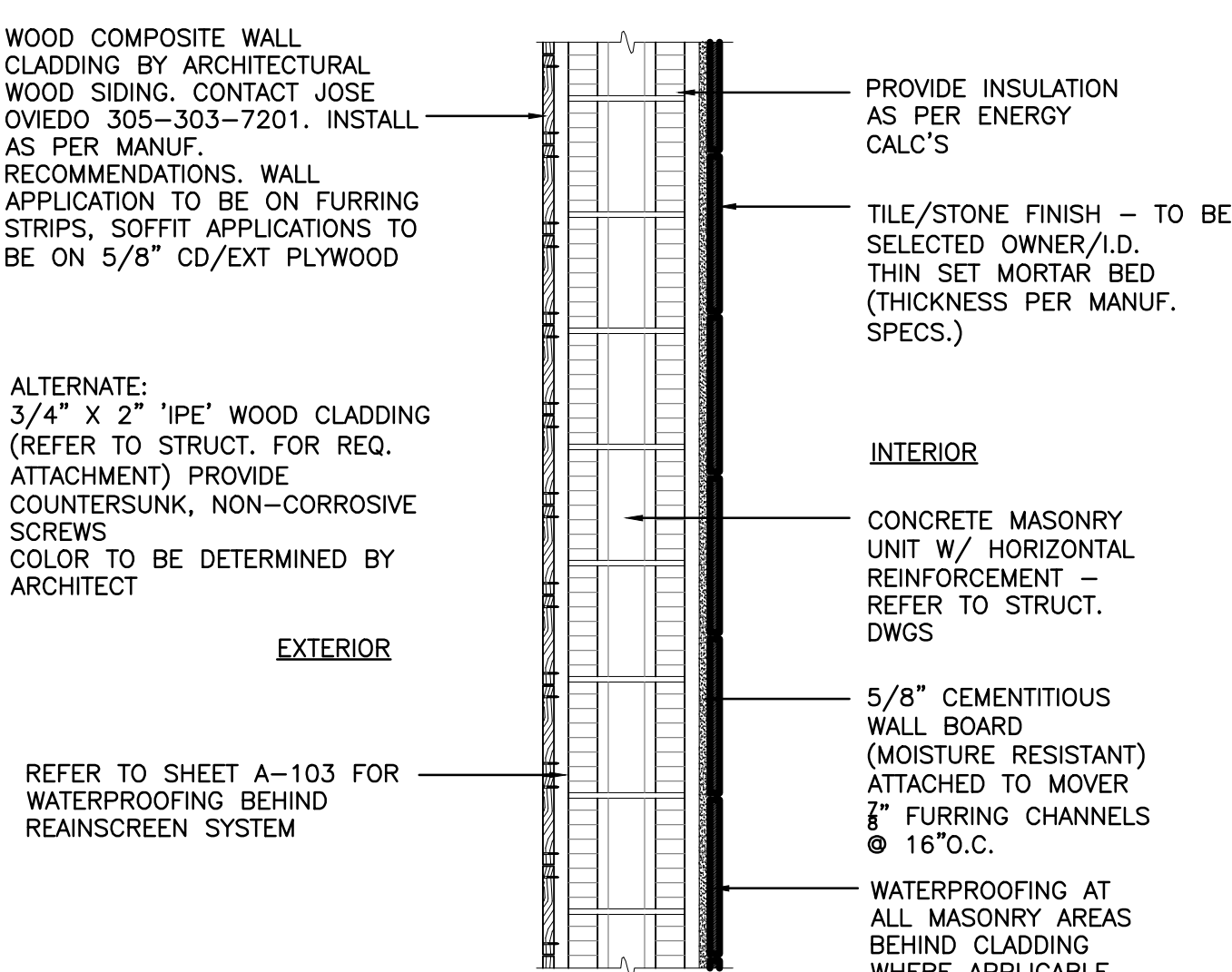
7 A-602 MASONRY - M7 SCALE: 1"=1'-0"
