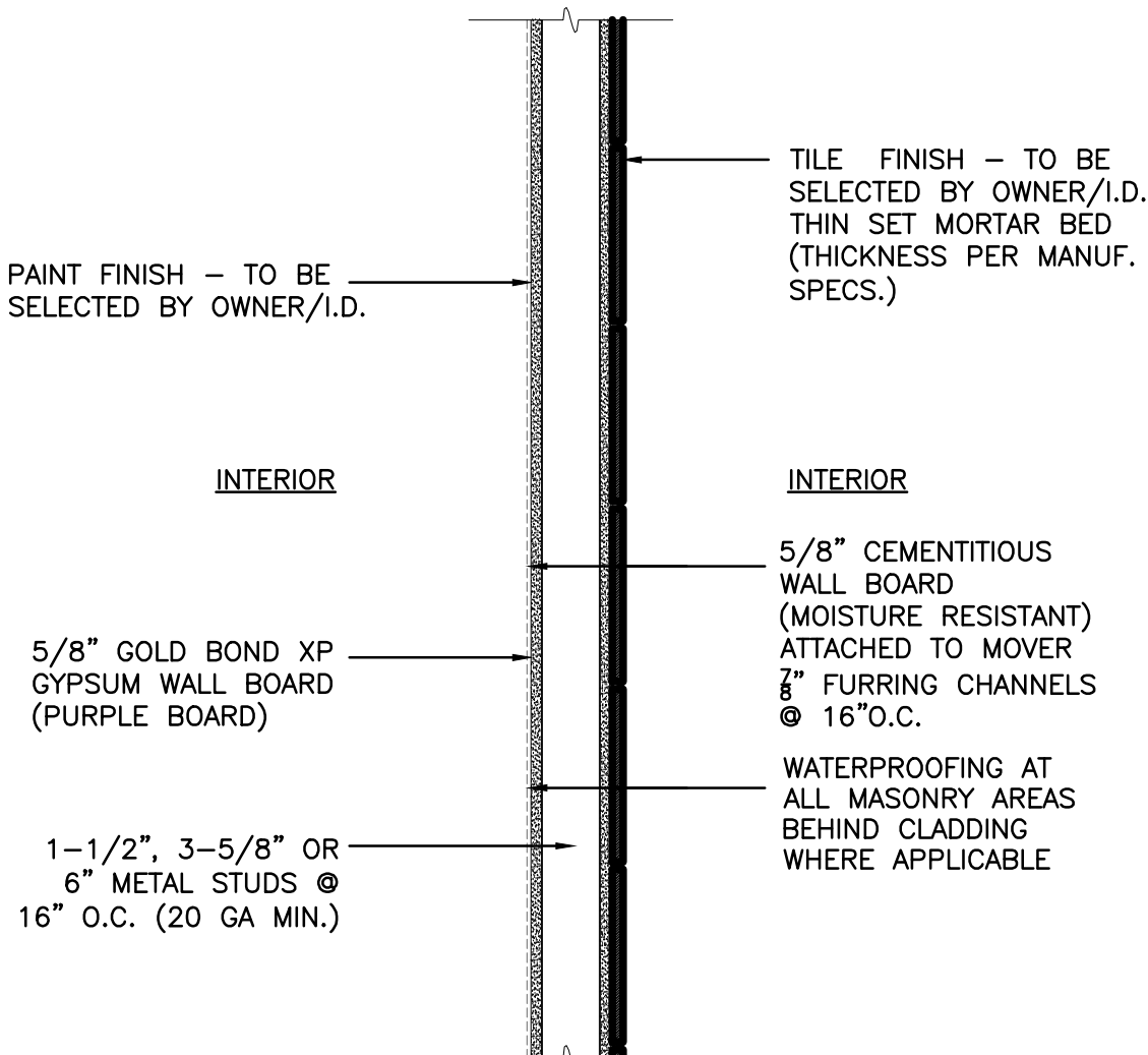
11 A-602 PARTITION - P2 SCALE: 1"=1'-0"
