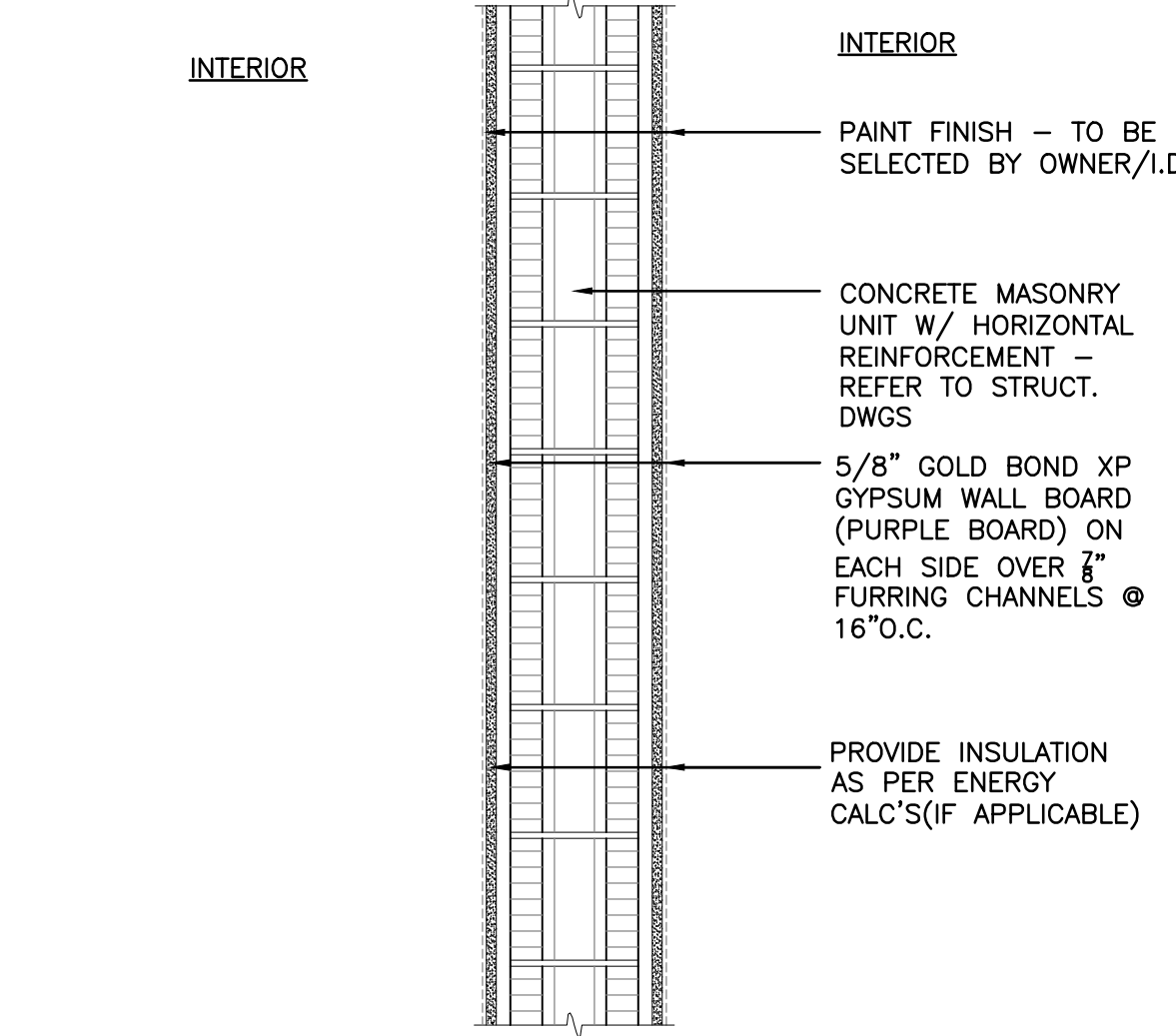
2 A-602 MASONRY - M2 SCALE: 1"=1'-0"
