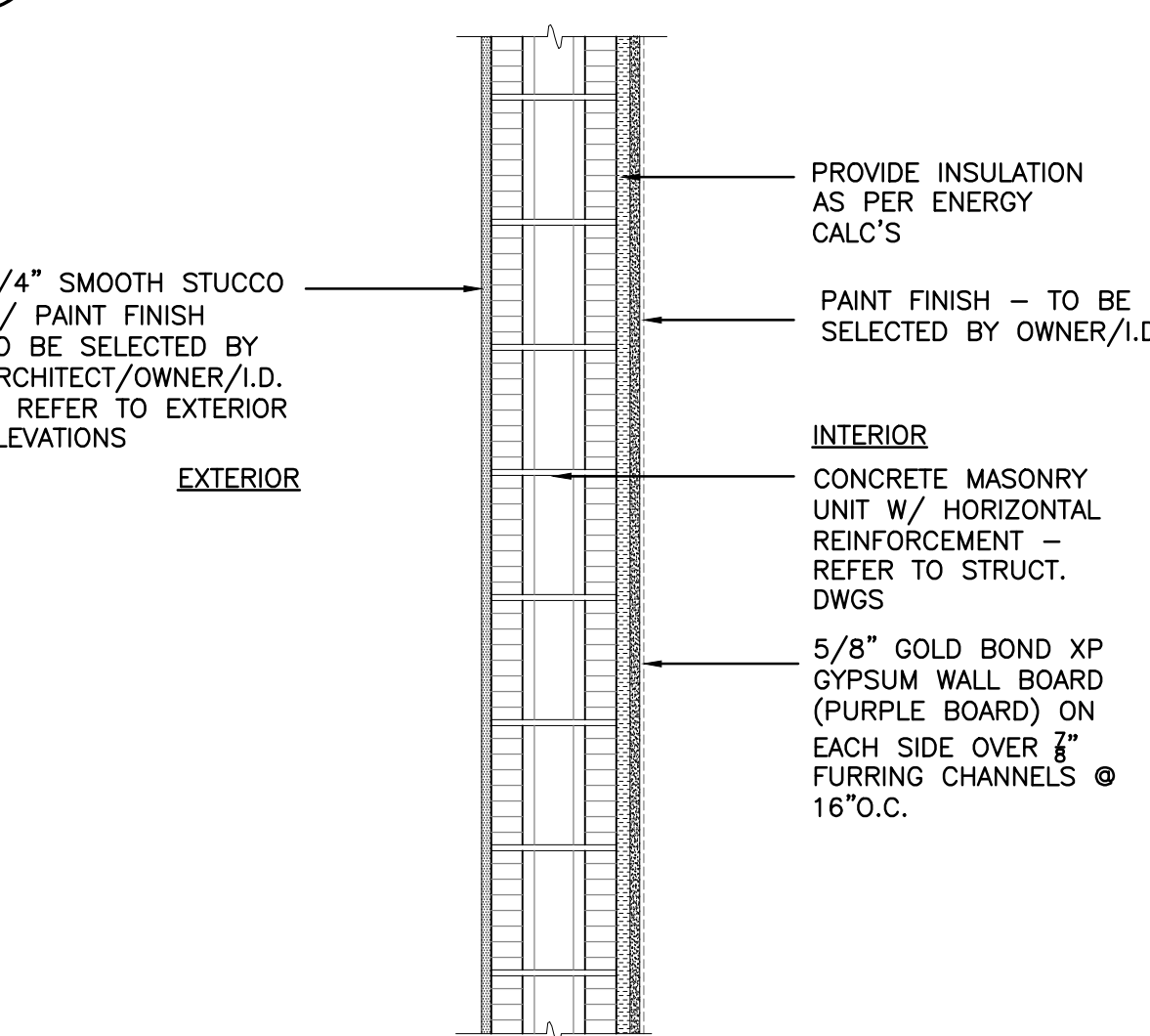
1 A-602 MASONRY - M1 SCALE: 1"=1'-0"
